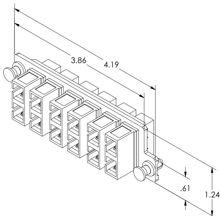
Ejemplo 6 x SC Duplex (Medidas en Pulgadas)
